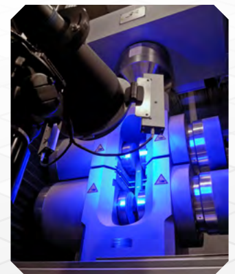
Extensomètre vidéo
