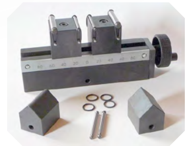
Outillages pour essais de flexion
